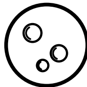
Ganymede
