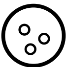
Io
